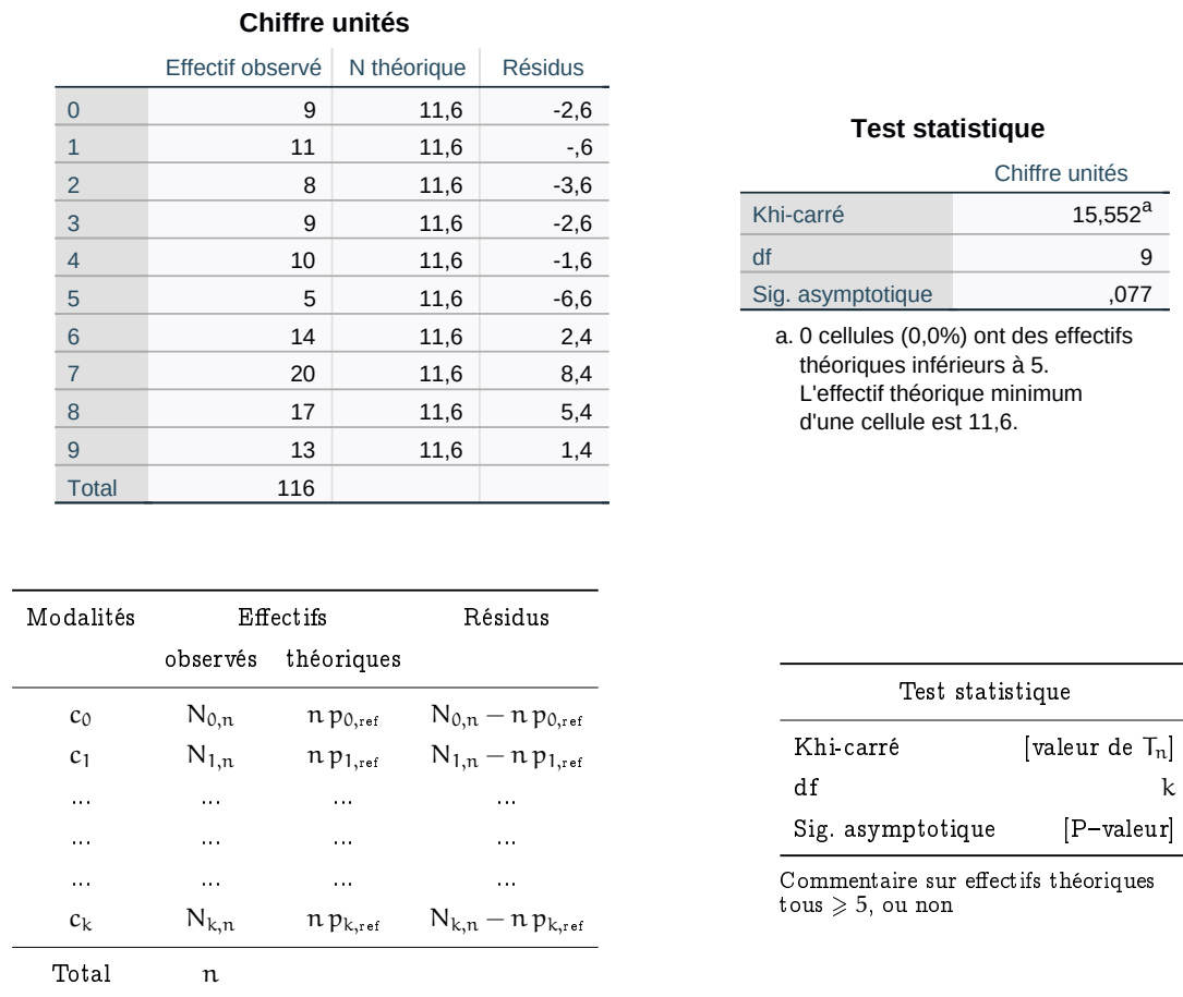
FIGURE 6.3 – Sortie logiciel [haut] correspondant à la mise en œuvre sur les données de la Figure 6.1 du test du \chi^2 d'ajustement à la loi uniforme sur \{0, 1, \dots, 9\} , et explication stylisée [bas] du contenu des tableaux.
